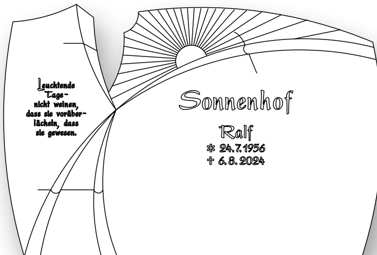
Breit STEIN
